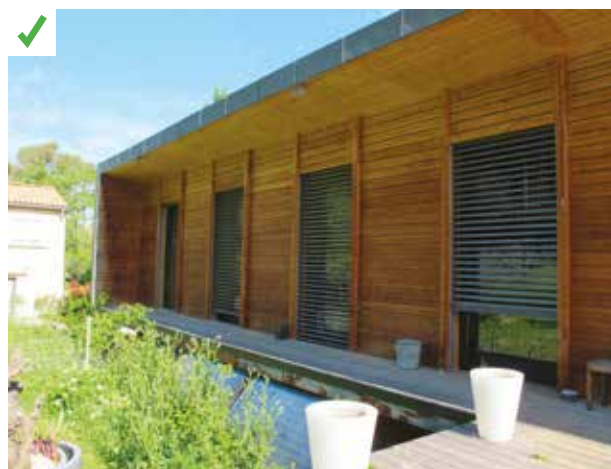
Brise soleil orientables (BSO) positionnés à l'extérieur et contribuant, en complément de la casquette correctement dimensionnée, à éviter les surchauffes et l'éblouissement en été sur la façade sud. ©AQC
